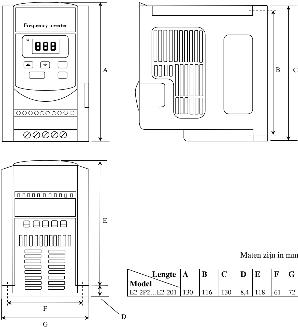
Fig. 1 Maatvoering E2 regelaars E2-2P2 t/m E2-201
