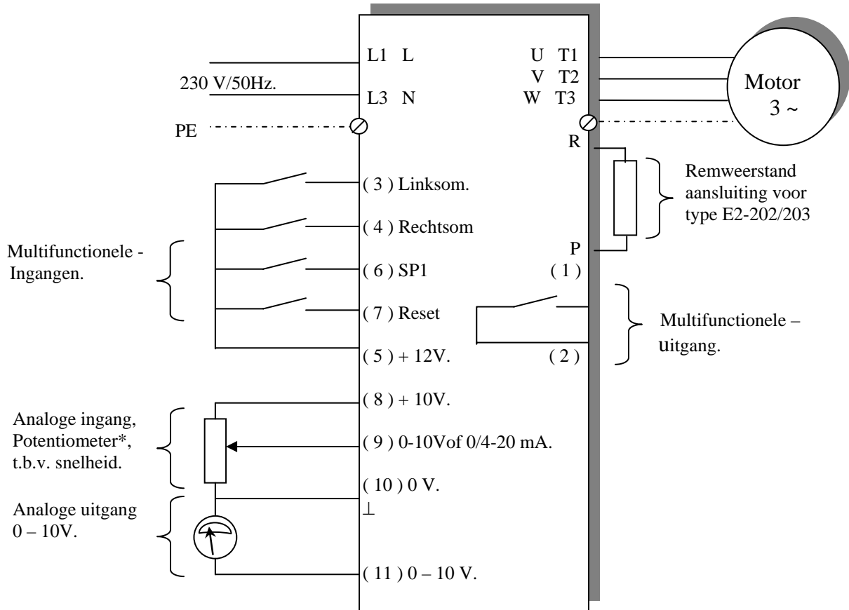
Fig. 9 aansluitschema E2 regelaar
