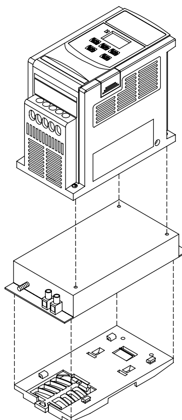
Fig. 5 Frequentieregelaar met klasse B filter en DIN montage
