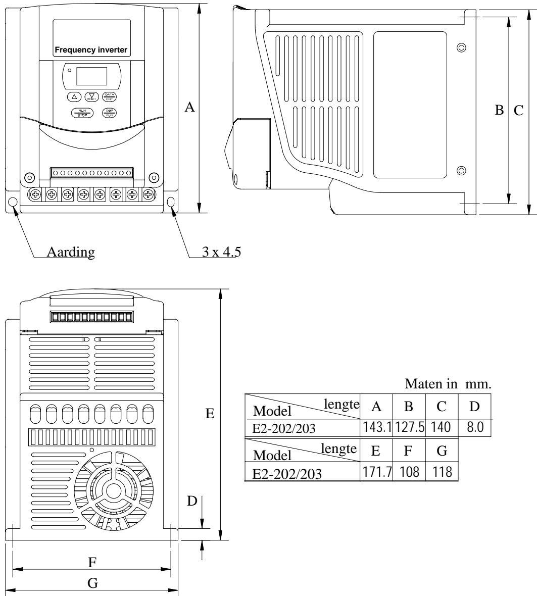
Fig. 2 Maatvoering E2-202-H1(F) t/m E2-203-H1(F)
