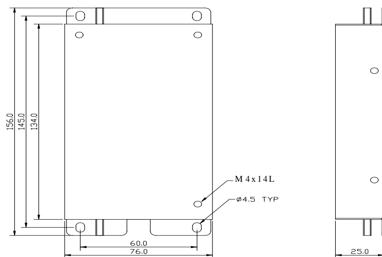
Fig. 3 afmetingen netfilter klasse B voor type E2-2P2-H1(F) t/m E2-201-H1(F)
