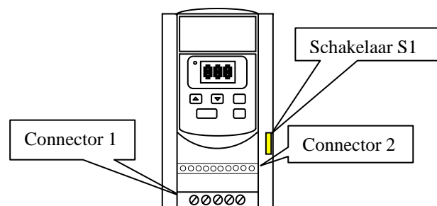
fig. 10 positie van de klemmenstroken op de E2 regelaar
